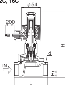
DP-12C, 16C
