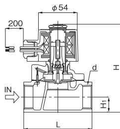
DP-16
