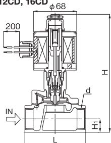
DP-12CD, 16CD
