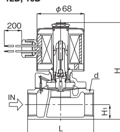
DP-12D, 16D
